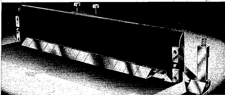
SECTIONAL CHIPBREAKER
